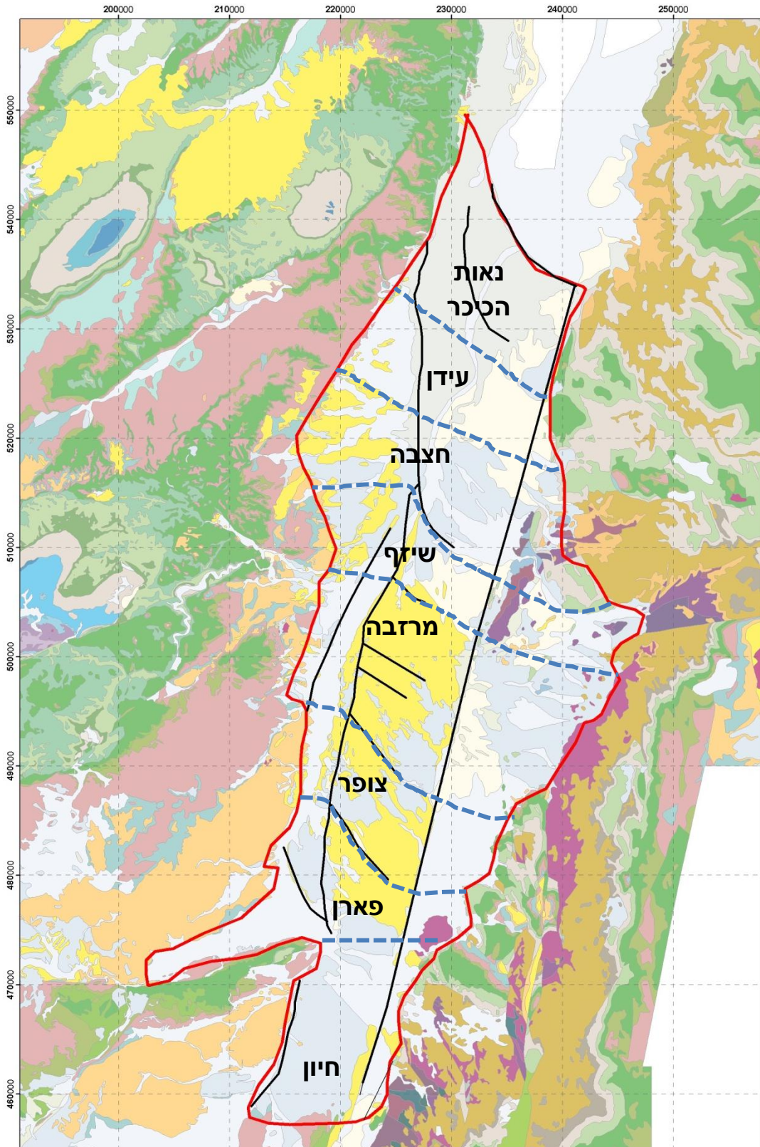
תרשים 1: גבול כללי של העבודה על בסיס תאי דיווח 751-752, על רקע מפה גיאולוגית, העתקים מרכזיים וחלוקה ראשונית משוערת ולא פרטנית לתאי משנה.
